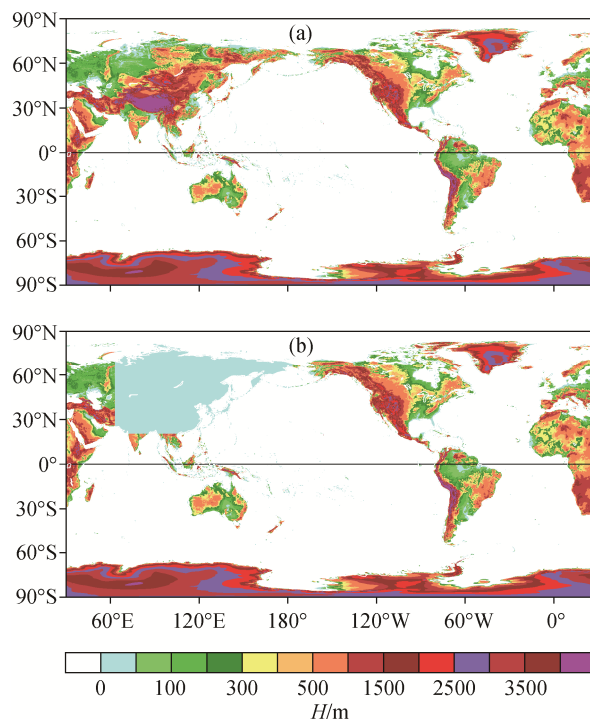
(a) Real 试验地形; (b) NoTibet 试验地形
