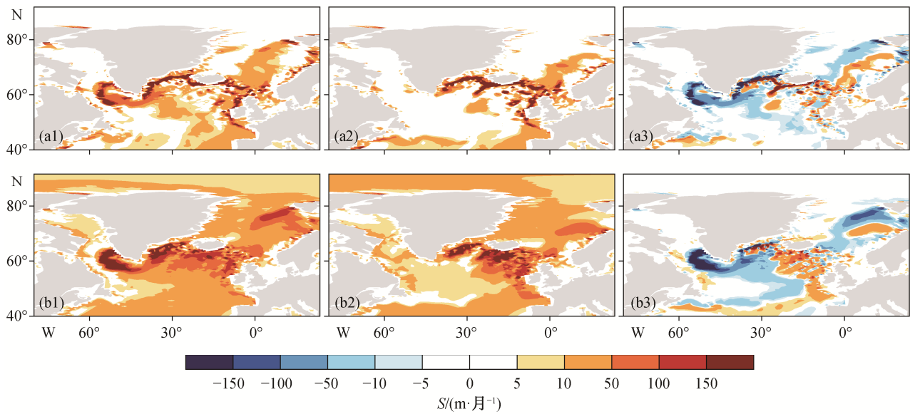
图 3 HR 试验中瞬时潜沉速率的水平分布 Fig. 3 Instantaneous subduction rate in the HR test
