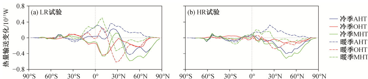
图 7 经向热量输送变化
