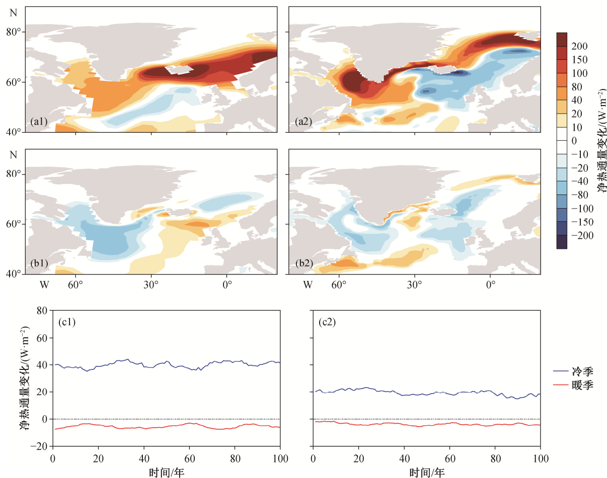
(a1)~(c1) LR 试验, (a2)~(c2) HR 试验; (a1)和(a2) 冷季海表净热通量变化, (b1)和(b2) 暖季海表净热通量变化, 正值表示海表净获得能量, 负值表示海表净失去能量; (c1)和(c2) NADW 形成区域海表净热通量变化时间序列
