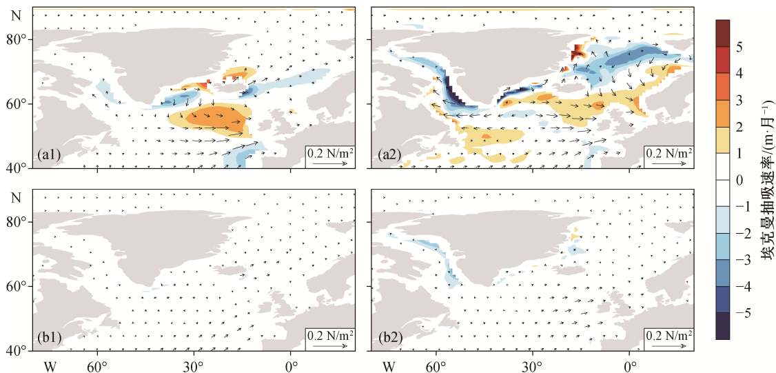
(a1)~(a2) 冷季, (b1)~(b2) 暖季; (a1)~(b1) LR 试验, (a2)~(b2) HR 试验。填色区域正值表示向上, 负值表示向下
