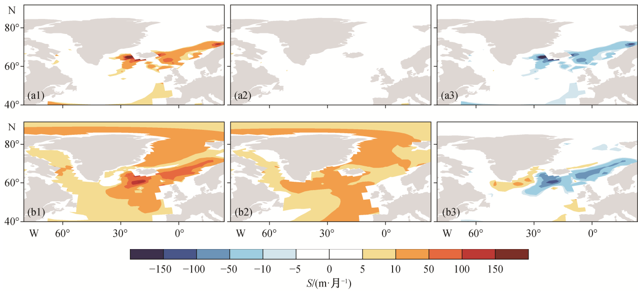
(a1)~(a3) 冷季试验, (b1)~(b3) 暖季试验; (a1)~(b1) Real 试验, (a2)~(b2) NoTibet 试验, (a3)~(b3) NoTibet 试验相对于 Real 试验的变化。为了更好地展示潜沉速率的空间分布, 将(a1)和(a2)及(b1)和(b2)中 S 负值设为 0。图 3 同
