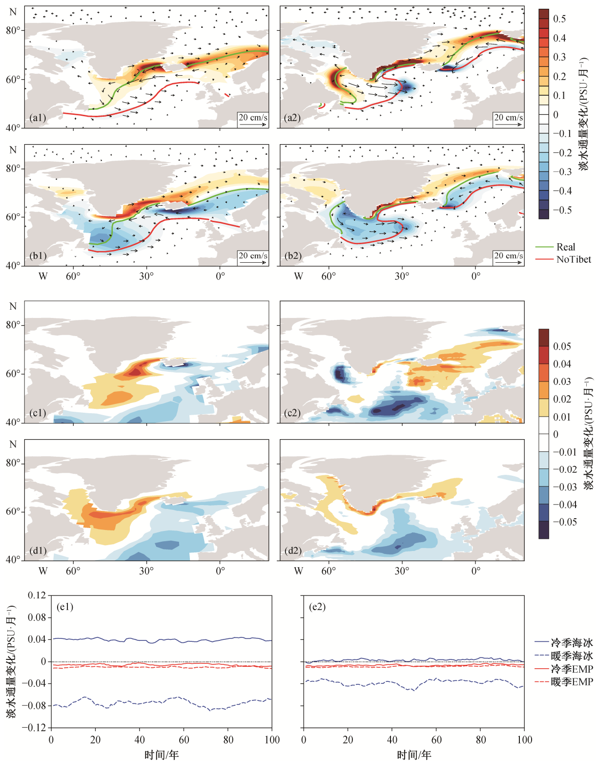
(a1)~(e1)LR 试验, (a2)~(e2)HR 试验; (a1)和(a2) 冷季海冰变化, (b1)和(b2) 暖季海冰变化, 包括海冰生消(填色区域正值表示海冰生成, 负值表示海冰融化、海冰移动速度变化(矢量箭头)和海冰边界变化); (c1)和(c2) 冷季 EMP 变化; (d1)和(d2) 暖季 EMP 变化, 正值表示海表失去淡水, 负值表示海表获得淡水; (e1)和(e2) NADW 形成区域淡水通量变化的时间序列
